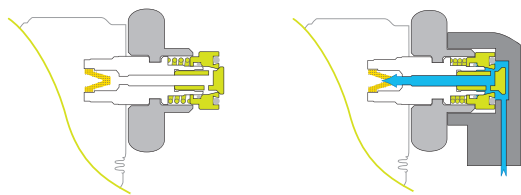
Регулятор отсоединен от вентиля > коннектор DIN закрыт
